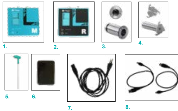
1. Meax LM 201 2. Meax LR 201 3. Spindelhållardiameter 16, 2 st. 4. Insatshylsa C25-16, 2 st. 5. Insexnyckel 6. Strömförsörjning, 4 USB-portar, 5 V DC 7. Extern strömkabel EUR 2 m 8. USB-kabel A-mini 0,5 m svart, 2 st.
